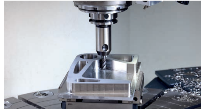
Nástroj: VHM stopková fréza Ø 10 mm
